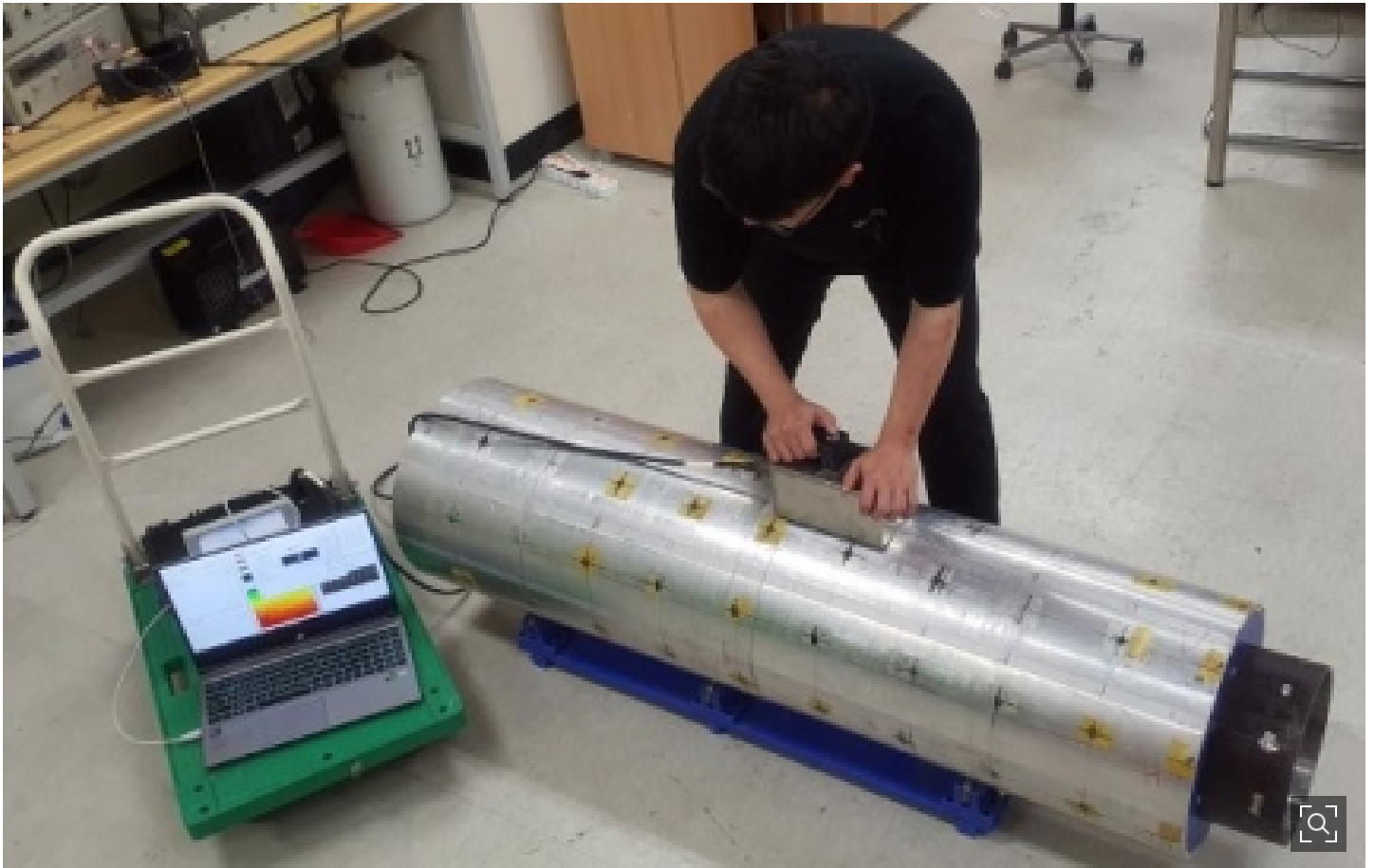
'보온재 비해체식 배관손상 평가기술'로 보온재를 해체하지 않고 배관 속을 검사한다. 원자력연구원 제공
